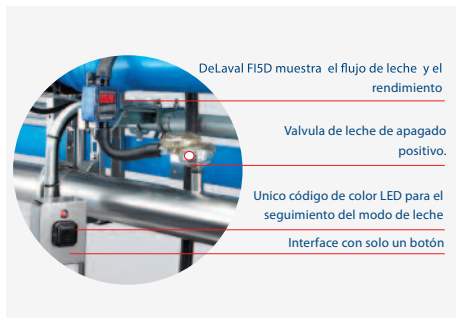
DeLaval MPC150B con DeLaval Fi7 indicador de flujo
